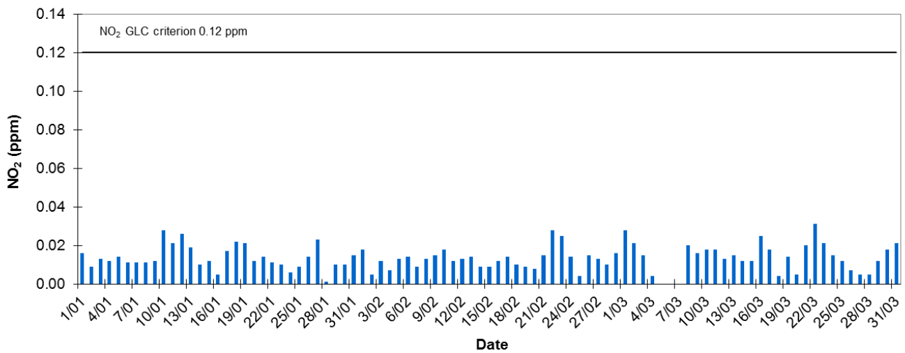
Le Fevre 2 1 Hr Daily Maxima NO2 - Quarter 1, 2016
