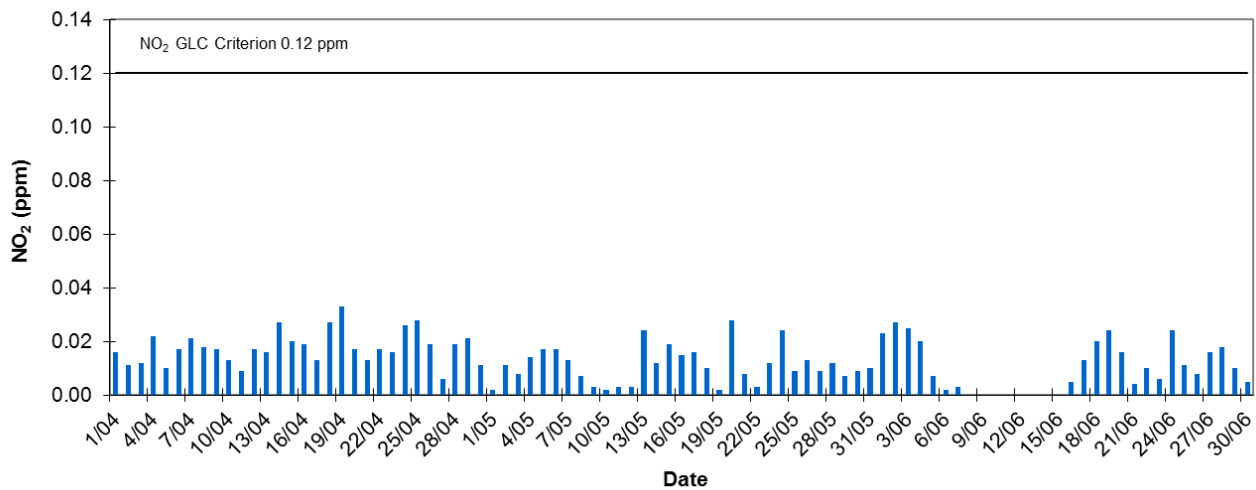
Le Fevre 2 1 Hr Daily Maxima NO2 - Quarter 2, 2016
