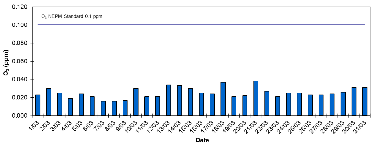
Le Fevre 2 1 Hr Daily Maxima O3 - March 2015
