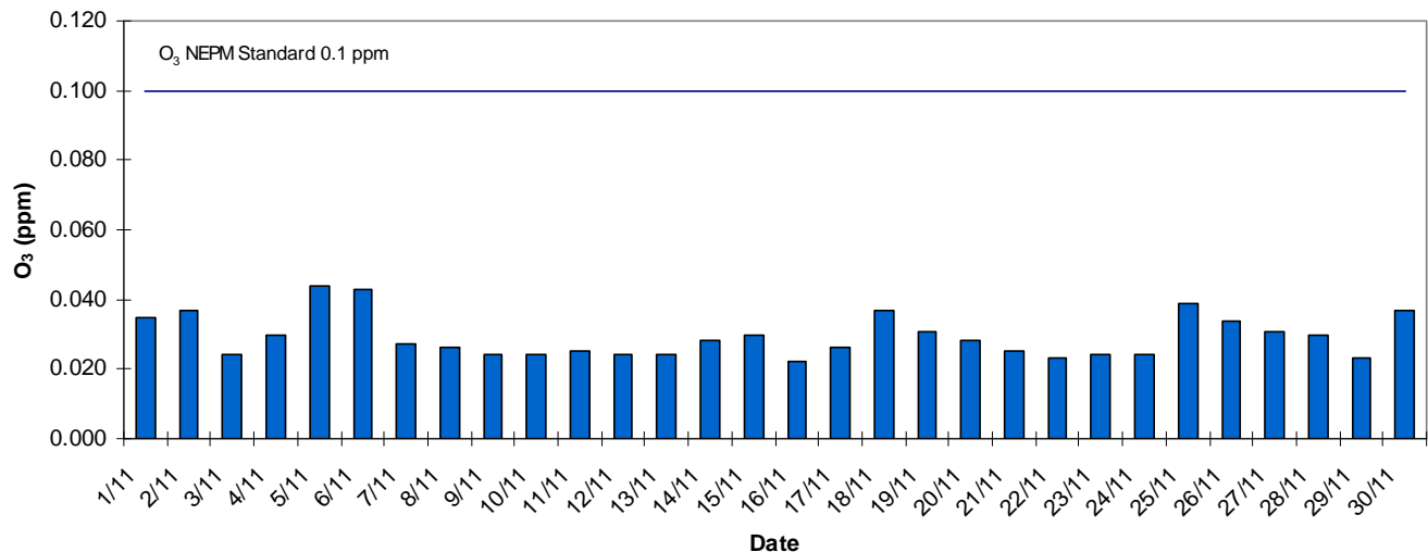
Le Fevre 2 1 Hr Daily Maxima O3 - November 2013
